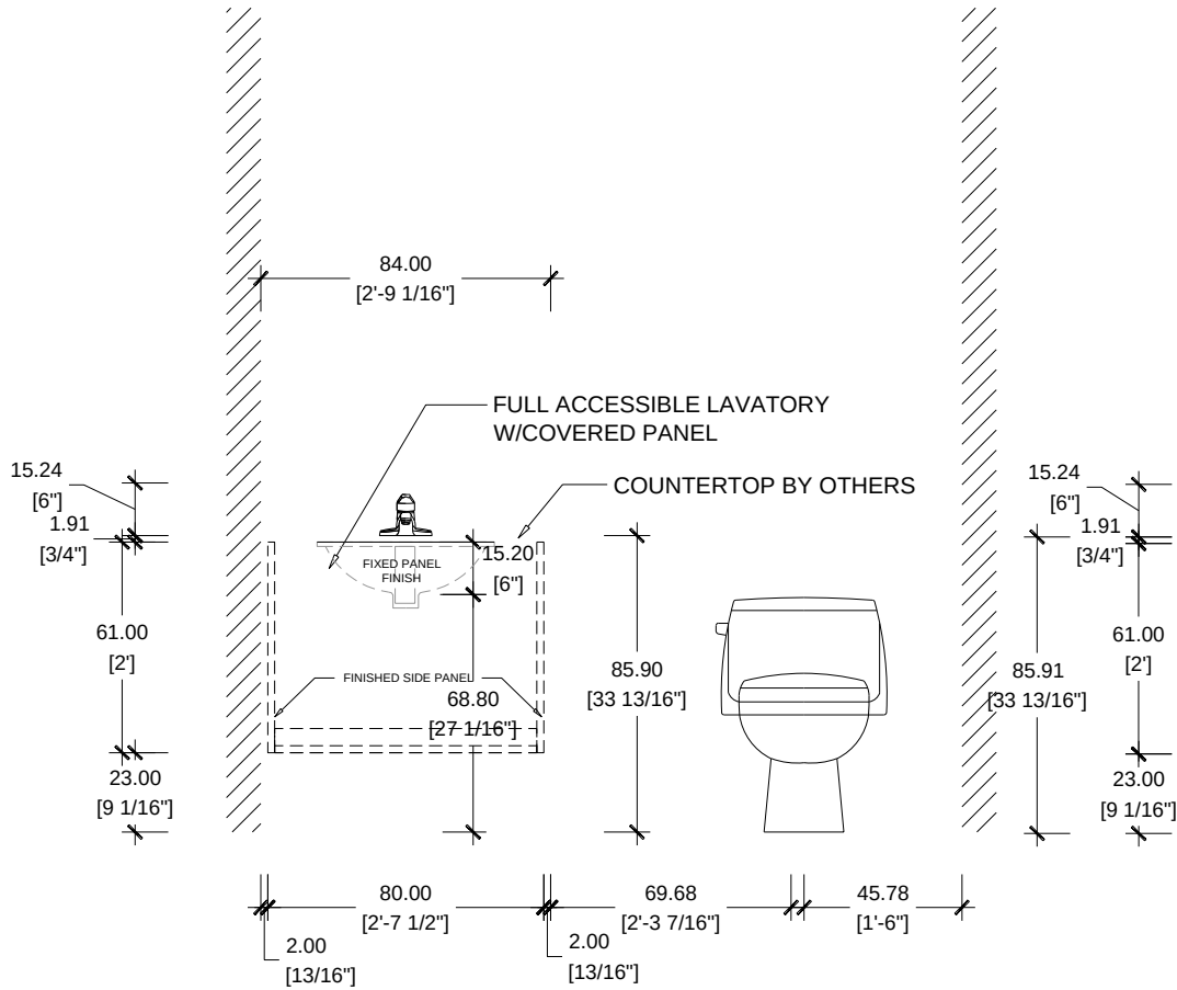
ELEVATION A CASA FAMILIA UNIT A2 FA / VANITY TYPE V2
